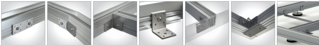
Profilverlängerung Variable Winkelverbindung Winkelverbindung Ballastaufnahme Verblendifixierung Winkelverstärkung Abstandshalter
